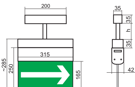
PROFIL - ceiling
